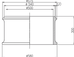
6 S-RB50(C)300
