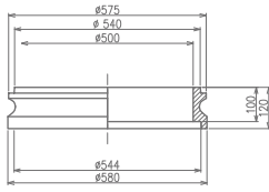
2 S-RB50(B)100
