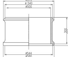
4 S-RB50(B)300
