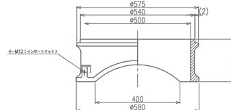
8 S-RB50(CTK)200M12
