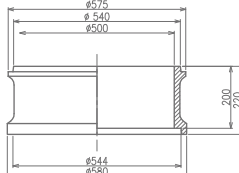
3 S-RB50(B)200
