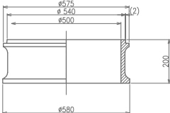
5 S-RB50(C)200
